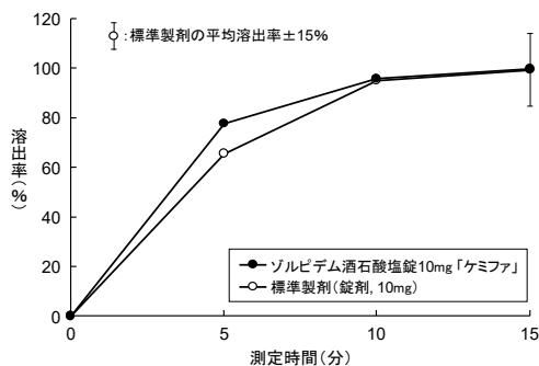
⑤水 (パドル法 50rpm)
