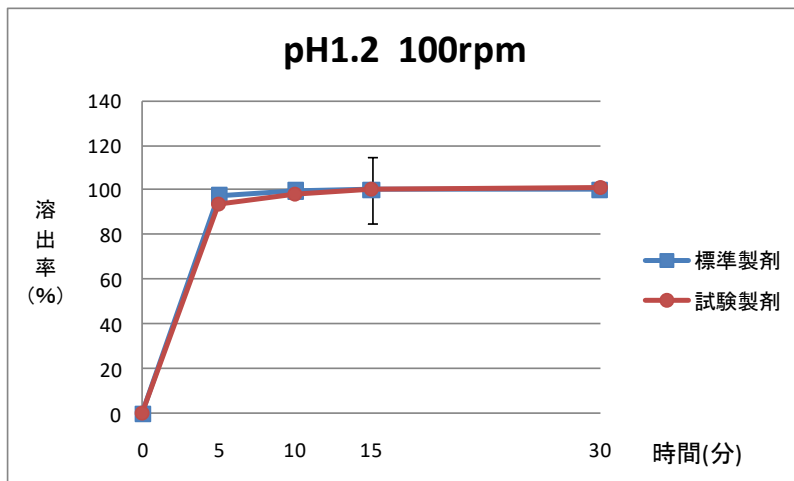
図 5：pH1.2 (100rpm)における溶出曲線
