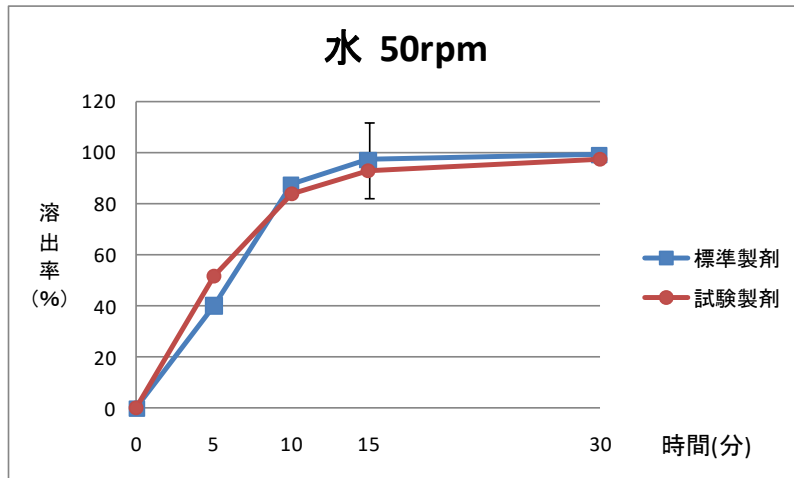
図 4：水 (50rpm)における溶出曲線
