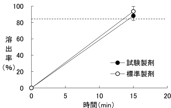
pH1.2における溶出曲線
